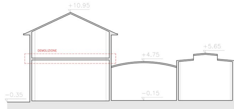
SEZIONE STATO DI FATTO
