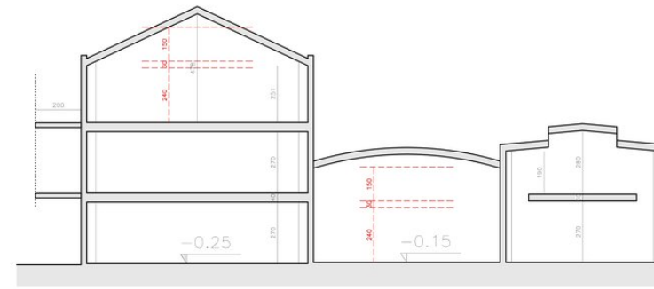
SEZIONE PROPOSTA DI MASSIMA
