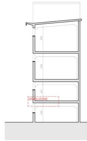
SEZIONE STATO DI FATTO
