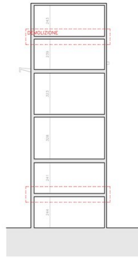
SEZIONE STATO DI FATTO
