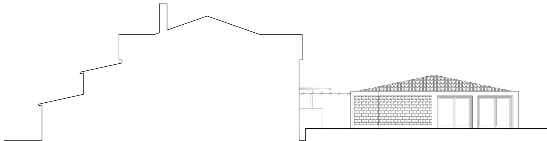
PROSPETTO SUD-OVEST
